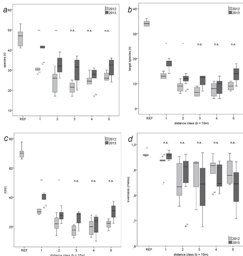
Slika 6: Spremembe v številu vrst (a), številu ciljnih vrst (b), podobnosti (FPFI) do ciljne površine (c) in izenačenosti (d) med petimi razredi oddaljenosti (širina razreda = 10 m) na nekdanji obdelovani površini med letoma 2012 in 2013. Spremembe smo primerjali za vsak dejavnik in razred oddaljenosti z z Mann-Whitney-evim- U testom (označeno z zvezdico ali z 'n.s.'). V tem primeru se obnovljene in primerjalna površina statistično značilno razlikujejo v vseh dejavnikih v vseh razredih oddaljenosti in letih ( p < 0,05 ). Edina izjema je izenačenost, ki se ne razlikuje med ciljno površino in razredih oddaljenosti 1(2013), 3(2013) in 5(2012) na obnovljenih površinah ( p \leq 0,05 ). n.s.: not significant ( p > 0,05 ), *: 0,01 < p \leq 0,05 , **: p \leq 0,01 .
