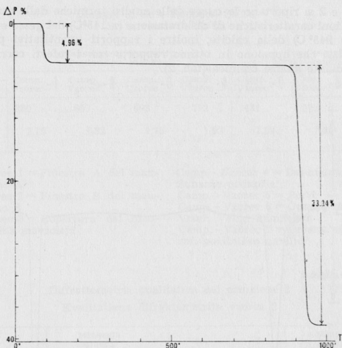
Fig. 2. Curva della analisi termodifferenziale Sl. 2. Krivulja termično-diferencialnih analiz
