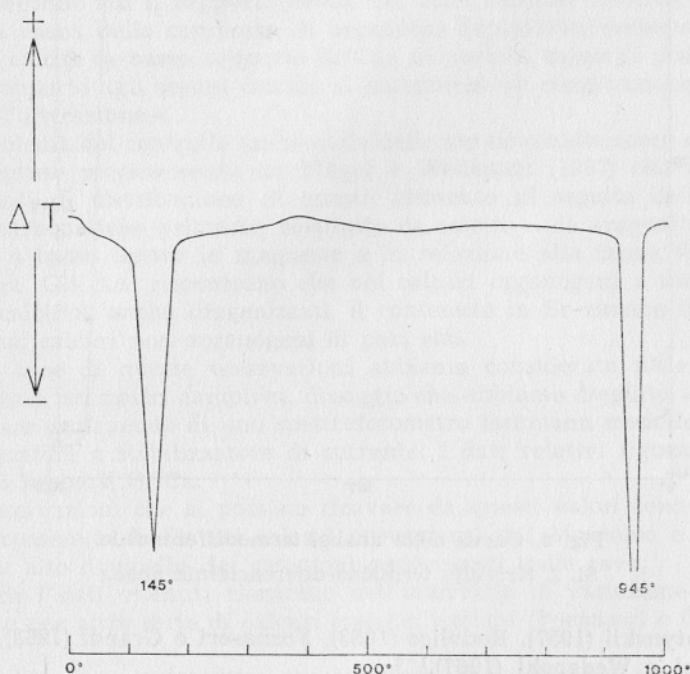
Fig. 1. Curva della analisi termoponderale Sl. 1. Krivulja termoponderalnih analiz
