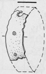
Koritnica. 1—3 železo, 4—6 bron Koritnica. 1—3 Eisen, 4—6 Bronze 1—6 = 1/2
