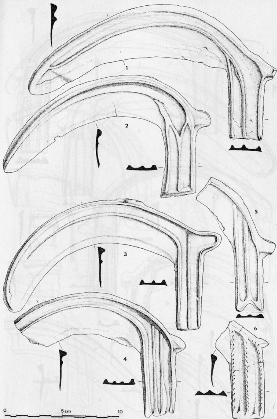
T. 3: Depojska najdba Debeli vrh nad Predgradom, vse bron. Pl. 3: The Debeli vrh depot above Predgrad, all bronze.
