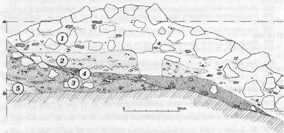
SI. 10: Martinj Hrib. Profila južne in vzhodne strani ruševin v sredini kvadranta 46. Abb. 10: Martinj Hrib. Profile der Süd- und Ostseite der Trümmer inmitten des Quadranten 46.
