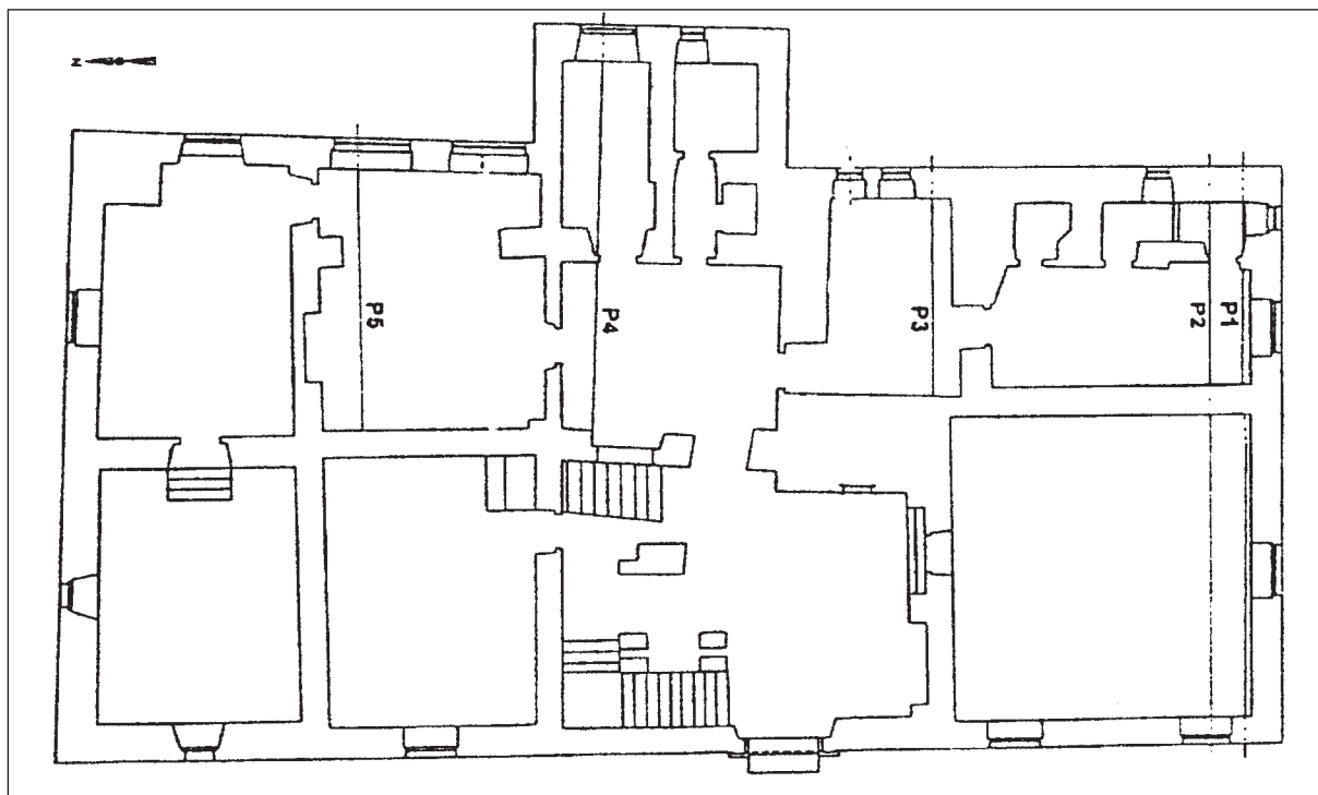
Sl. 7: Polhov Gradec-graščina. Tlorisni načrt predstavljenih prereзов. M. = 1:200. Fig. 7: Polhov Gradec-manor house. Plan of the presented cross-sections. Scale = 1:200.
