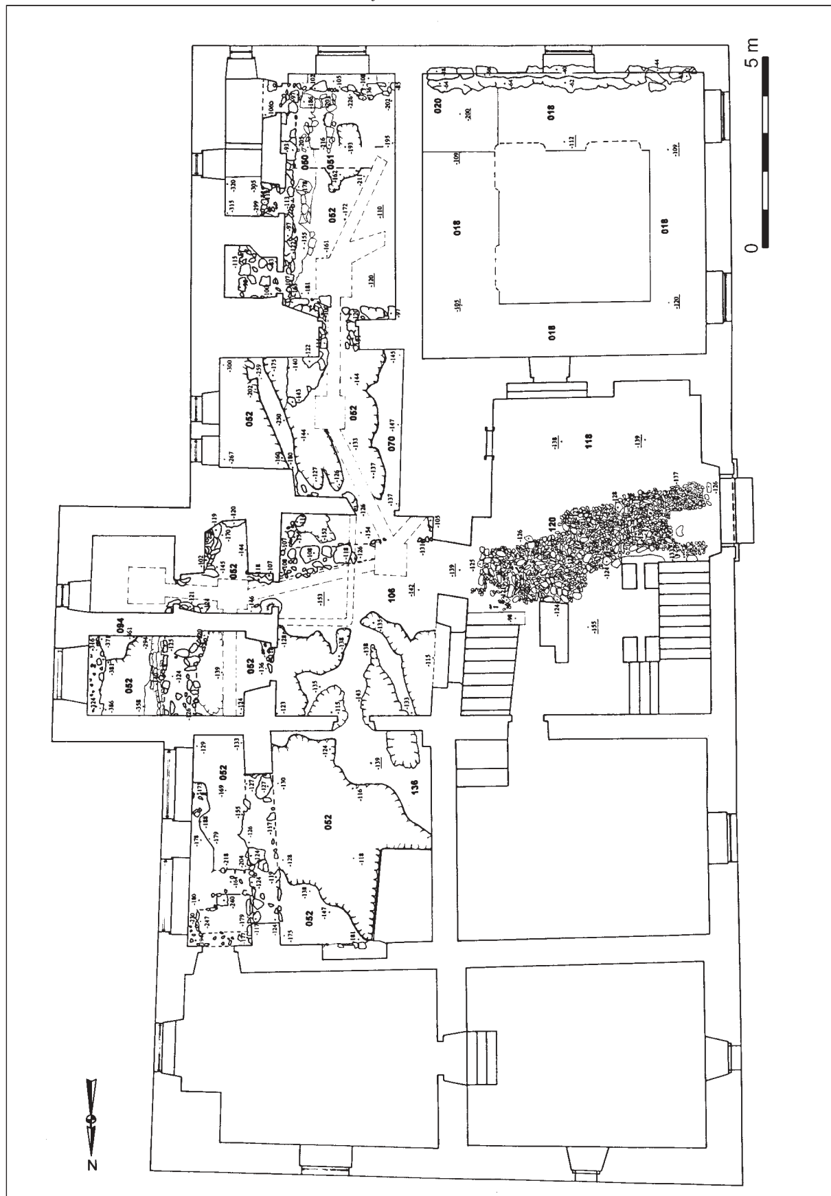
Sl. 6: Polhov Gradec-graščina. Torlis geološke osnove in starejših temeljev.
