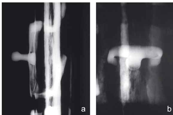
Sl. 5: Rentgenski posnetek zanke: a - s strani (90 KV, 4 mA, 1 min); b - z vrha, rahlo poševno (90 KV, 4 mA, 1 min).
