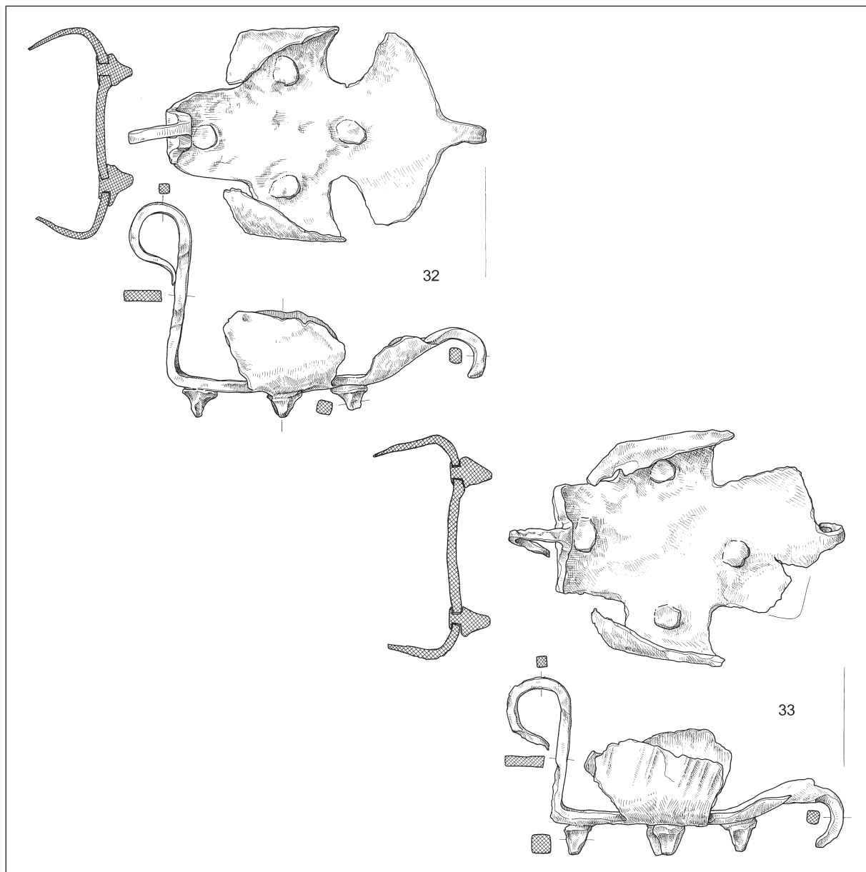
Fig. 14: Two hipposandals (32, 33) from Vodice. Iron. Scale = 1:3. Sl. 14: Dve obušvali kopit (32, 33) z Vodice. Železo. M. = 1:3.
