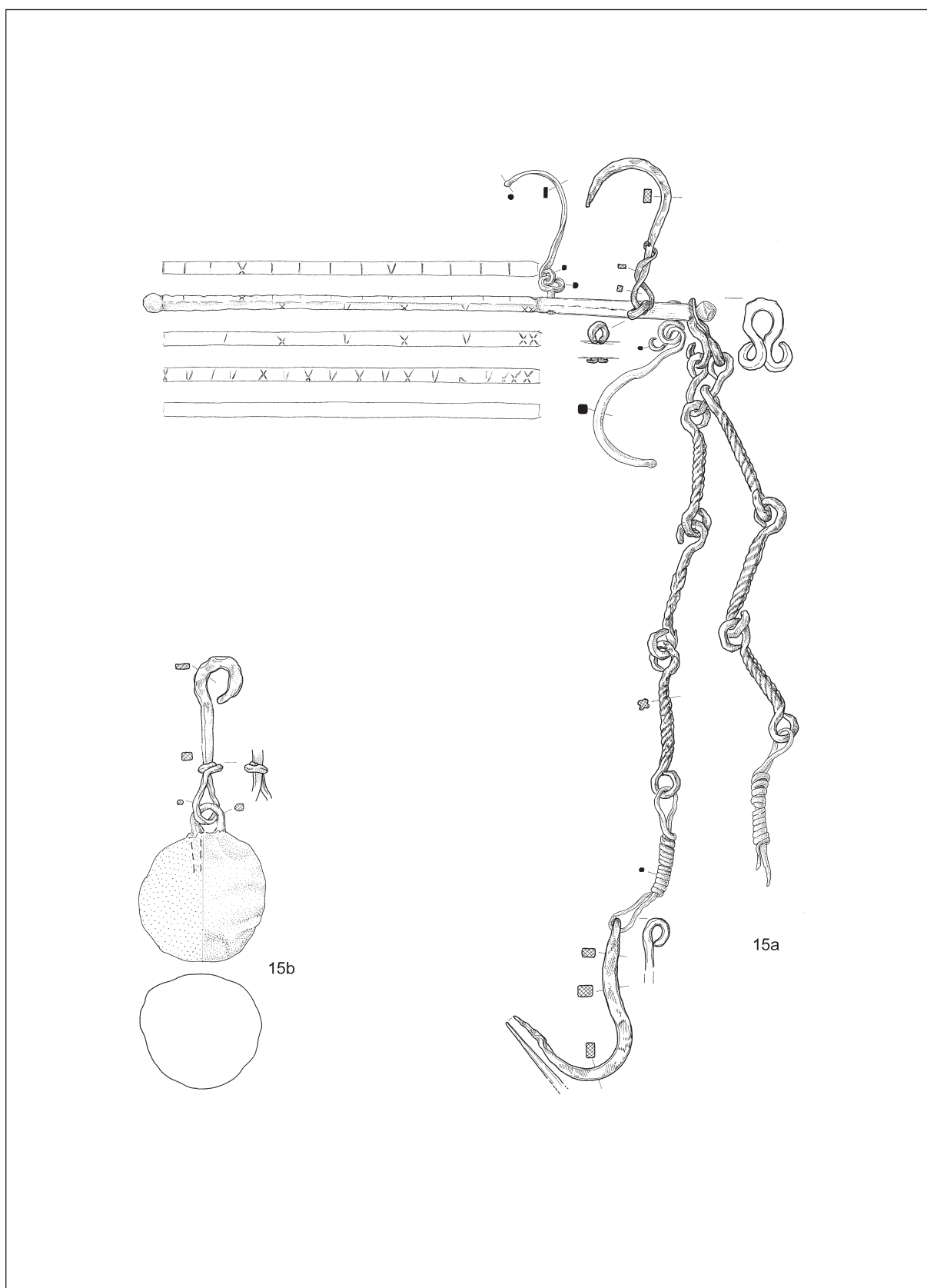
Pl. I: Vodice near Kalce, the supposed hoard. Steelyard (15) (Fig. II). Bronze, iron. Scale = 1:3. T. I: Vodice pri Kalcah, domnevna zakladna najdba. Tehnica (15) (sl. II). Bron, železo. M. = 1:3.
