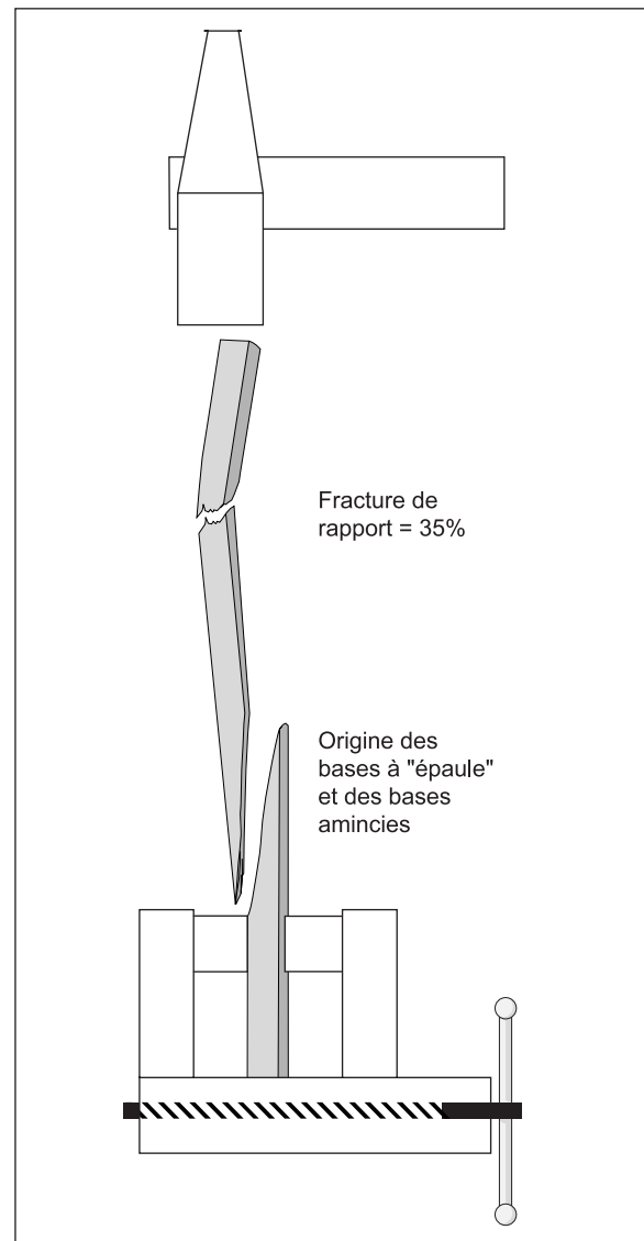
Fig. 3 Frappe au marteau: Baguette de sapin; section 2 × 6 mm 3 ; longueur 24 mm: Double fracture expérimentale: Encastrement dans un étau: La baguette doit toucher le fond: Explication de l'origine des bases à "épaule" d'Istállóskő et des bases amincies de certaines pointes de Potočka zijalka:
