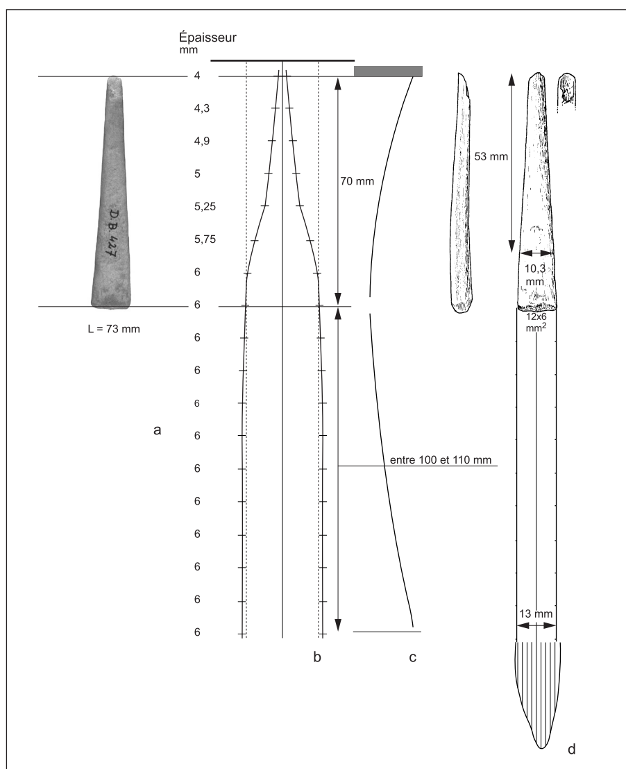
Fig. 7a-d: Pointe D: b: 538: La procédure complète de reconstruction: )a Face arrière de la pointe D: b: 538: )b Patron réalisé à partir du Tab: 3: )c Le flambage du patron découpé: La courbure maximale est proche du point de fracture terminale: )d La reconstruction de la partie proximale: Le résultat final après plusieurs retouches du patron: Échelle 3-4: Sl. 7a-d: Konica D. b. 427. Celoten postopek rekonstrukcije. (a) Zadnja stran konice D. b. 427. (b) Šablona narejena s pomočjo podatkov v tab. 2. (c) Obremenitev izrezane šablone in posledica obremenitve. Največji upogib je približno v predelu terminalnega preloma. (d) Rekonstrukcija proksimalnega dela. Končni rezultat na podlagi več popravkov šablone. 2/3 naravne velikosti.
