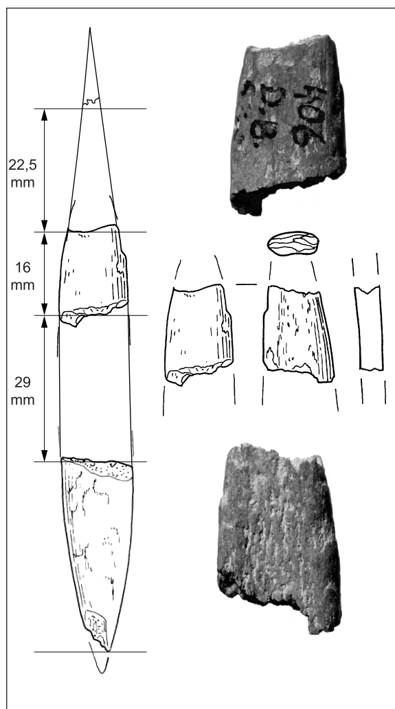
Fig. 13: Reconstruction du fragment D. b. 406 avec le fragment de base D. b. 7. Échelle 1 sauf photo : vue avant et arrière du fragment qui est à échelle 2. Longueur reconstruite 120,5 mm.
