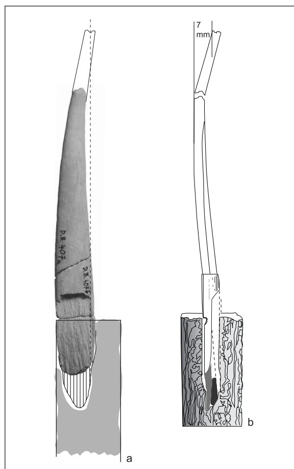
Fig. 5a,b: Pointe D. b: 5 8: )a Reconstruction avec emmanchement: Face extérieure avec la lèvre intérieure conservée: Allongement éventuel des lèvres: La fente se prolonge au moment de la flexion: )b Fixation par coin: Formation d'une "épaule" par la cassure: Échelle 3-4:
