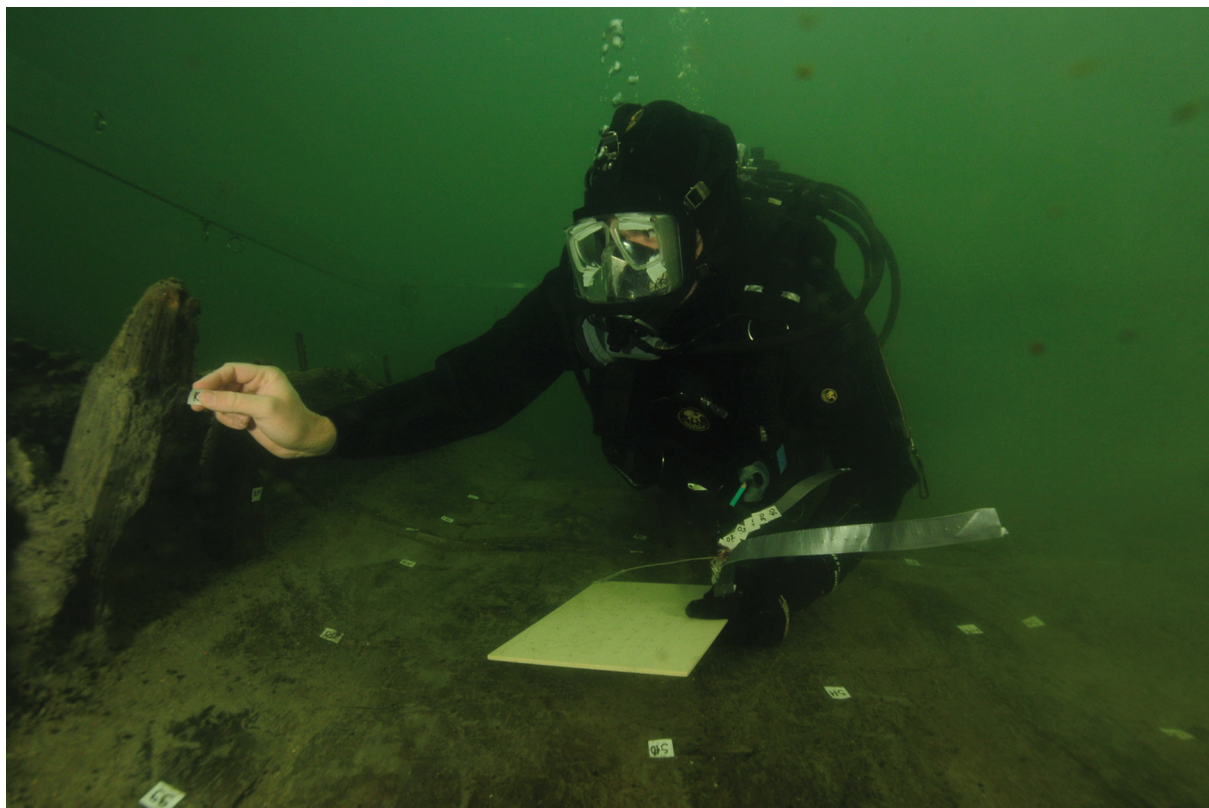
Sl. 3: Ljubljana pri Sinji Gorici. Označevanje elementov ladje za fotogrametrično 3R-modeliranje. Fig. 3: The Ljubljana at Sinja Gorica. Marking barge elements for photogrammetric 3D modelling. (Foto / Photo: R. Kovačič)
