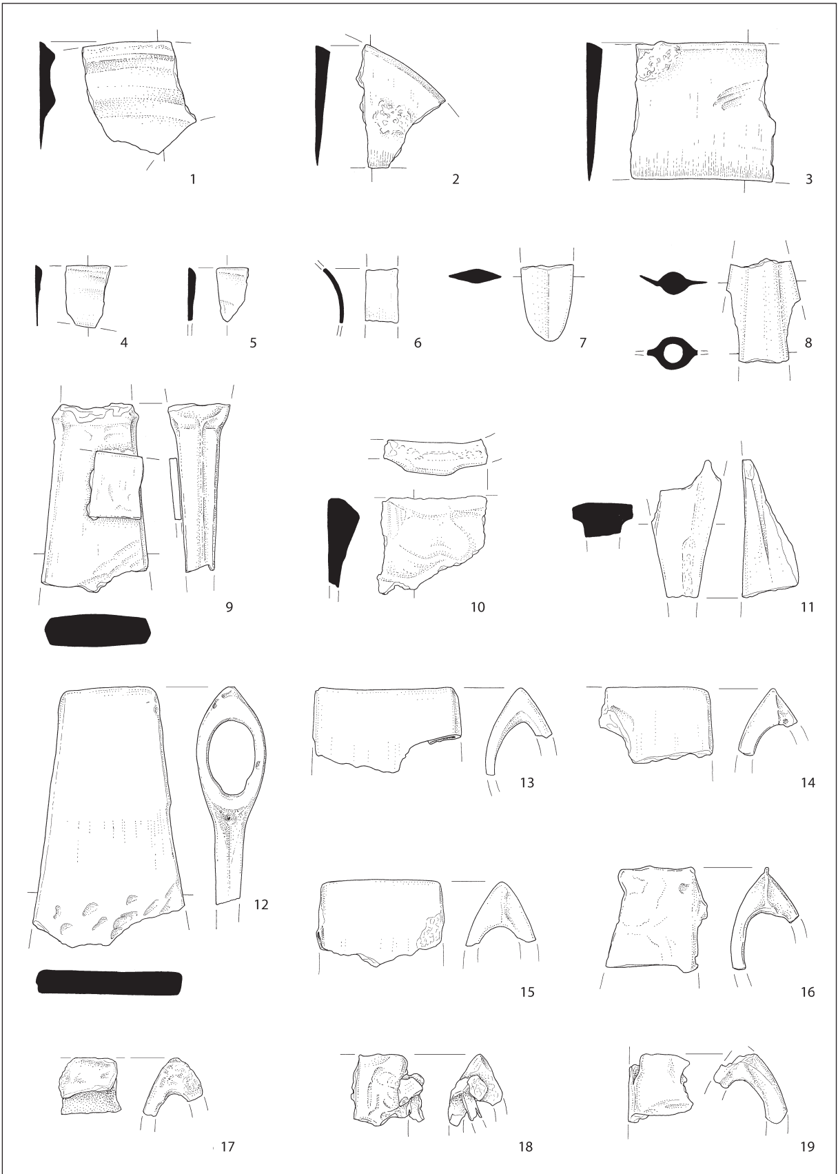
T. 1: Kranj – Jelenov klanec. Depo. Vse bron. M. = 1:2.
