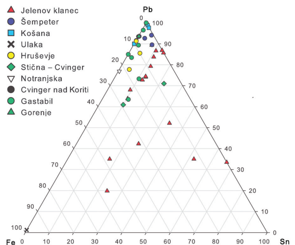
Sl. 22: Kranj – Jelenov klanec. Depo. Razmerje med kositrom, svincem in železom v uhatih sekirah.
