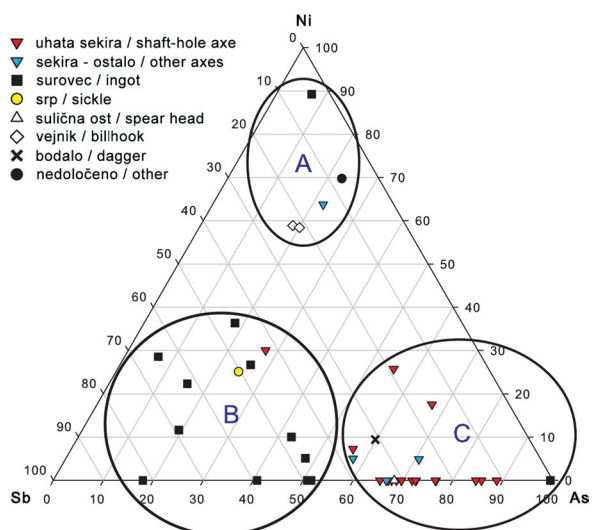
Sl. 17: Kranj – Jelenov klanec. Depo. Razmerje med arzenom, nikljem in antimonom v predmetih.
