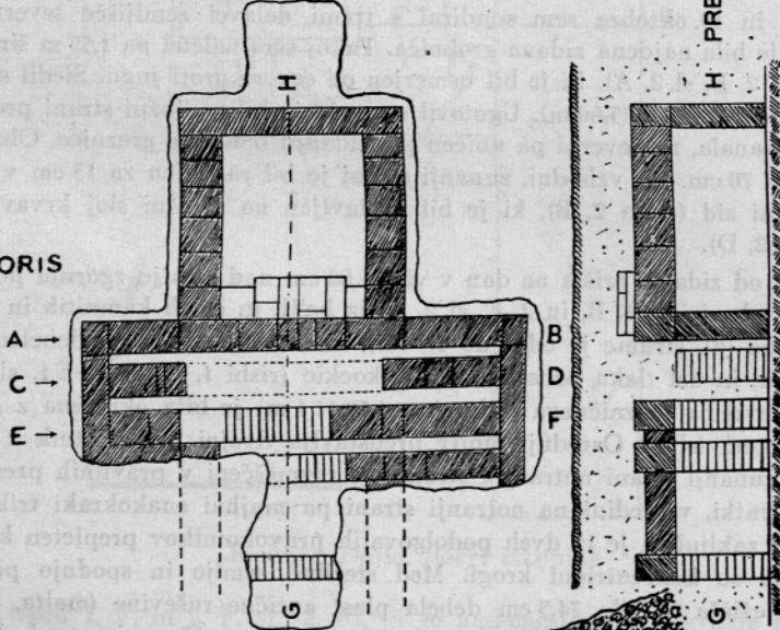
RIMSKA LONČARSKA PEČ PTUJ - PARCELA 196
