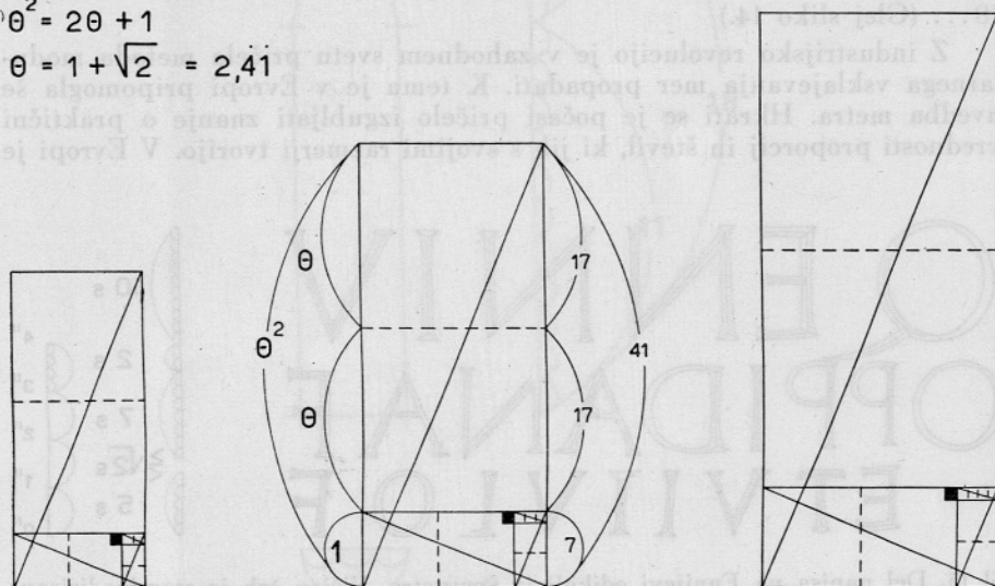
Sl. 12. Grafična predstava prvih treh Pellovih zaporedij, pri katerih razmerje med sosednjimi členi limitira k vrednosti \Theta = 1 + \sqrt{2} . Za našo razpravo je zanimivo drugo zaporedje s ključnim številom 7, torej 1 - 3 - 7 - 17 - 41 \dots
