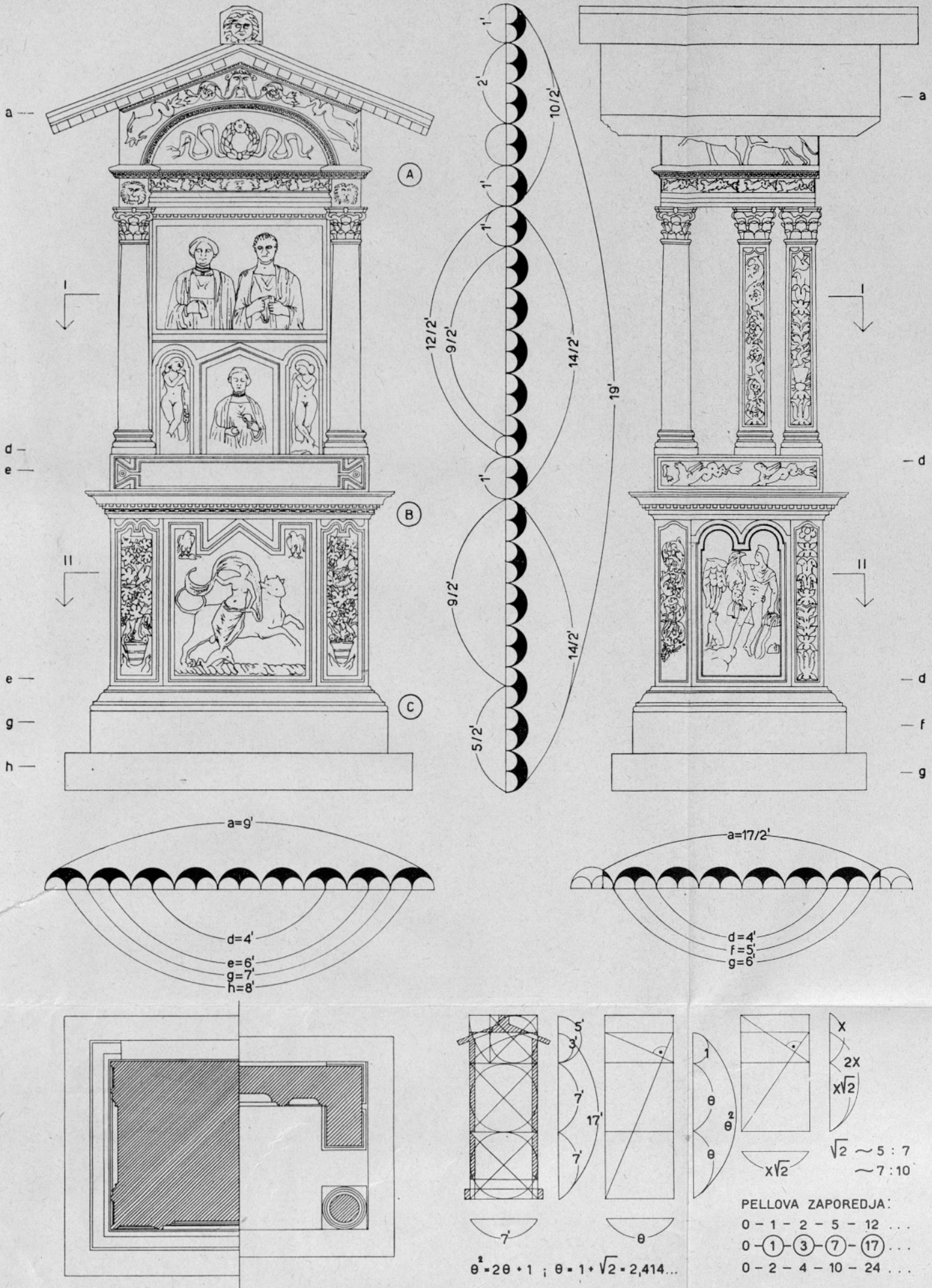
Sl. 11. Ennijeva edikula iz Šempetra. — Mere edikule in njenih členov so izrazljive z mnogokratniki rimskih čevljev. Mnogokratnik 7, ki določa višino podstavka, 7, ki določa visino srednjega dela edikule, in 5, ki določa višino zaključka, reduciranega na pravokotnik, so členi iz drugega Pellovega zaporedja 1 — 5 — 7 — 17...
