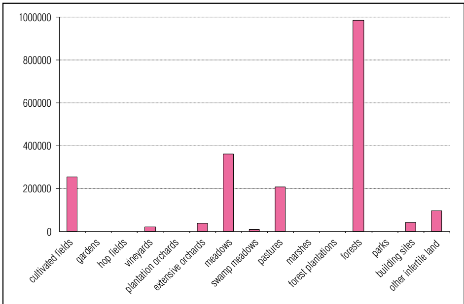
Figure 13: Surface Area of Cadastral Land Categories in Slovenia in 1991 (in hectares). Slika 13: Površina katastrskih zemljiških kategorij v Sloveniji leta 1991 (v ha).
